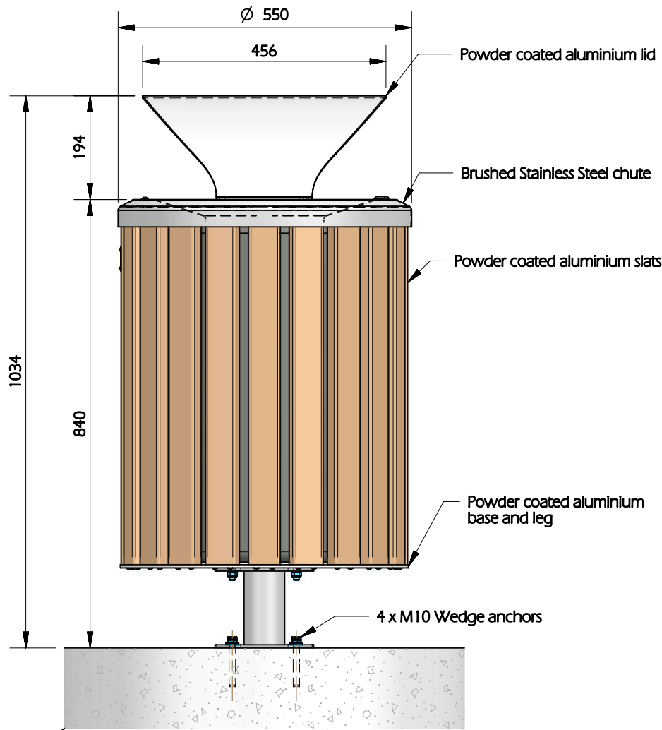
ELEVATION SCALE: NTS
