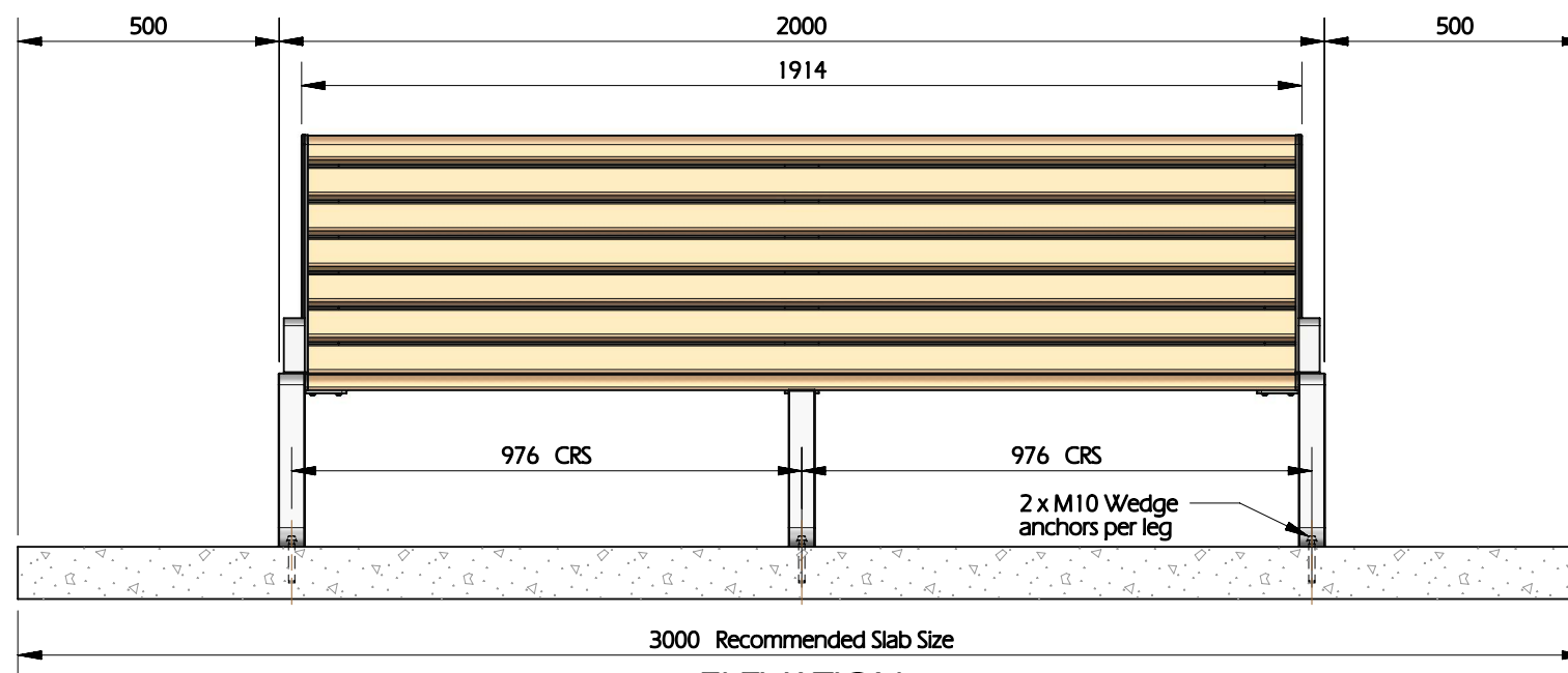
ELEVATION SCALE 1:15
